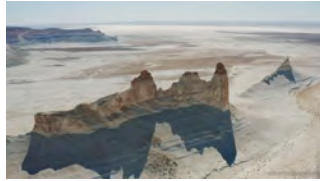
ウスチュルト台地
